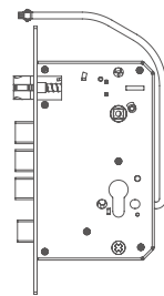
● 鎖匣
